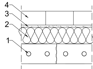
Rysunek 3.3. Ściana szczelinowa; 1 – blok Silka, 2 – izolacja, np. Multipor, 3 – pustka powietrzna, 4 – blok Silka, cegła Silka 1NF lub cegła klinkierowa
