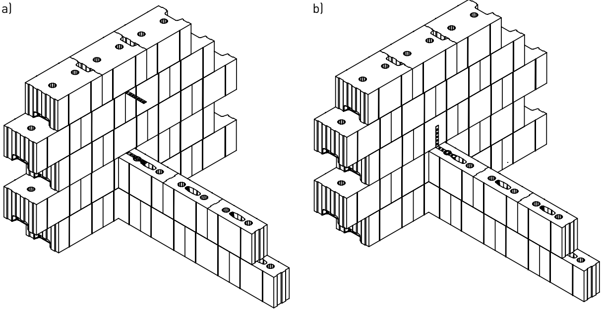
Rysunek 3.9. Łączenie ścian działowych usytuowanych prostopadłe. Ściany łączone na dotyk, kotwione za pomocą blach i kątowników: a) gdy położenie ścianek działowych jest znane w momencie murowania ścian nośnych b) gdy położenie ścianek działowych nie jest znane w momencie murowania ścian nośnych
