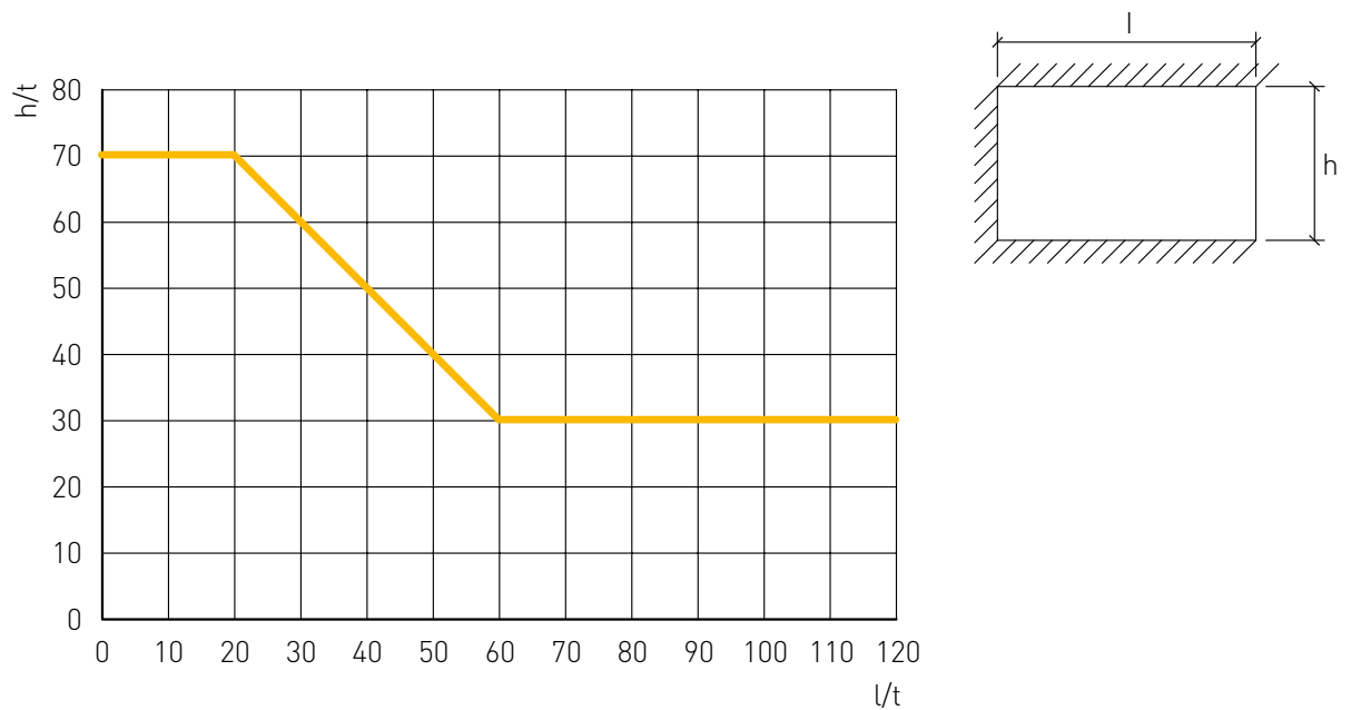
Wykres 3.2. Maksymalne wymiary ściany zamocowanej na trzech krawędziach: dolnej, górnej i bocznej
