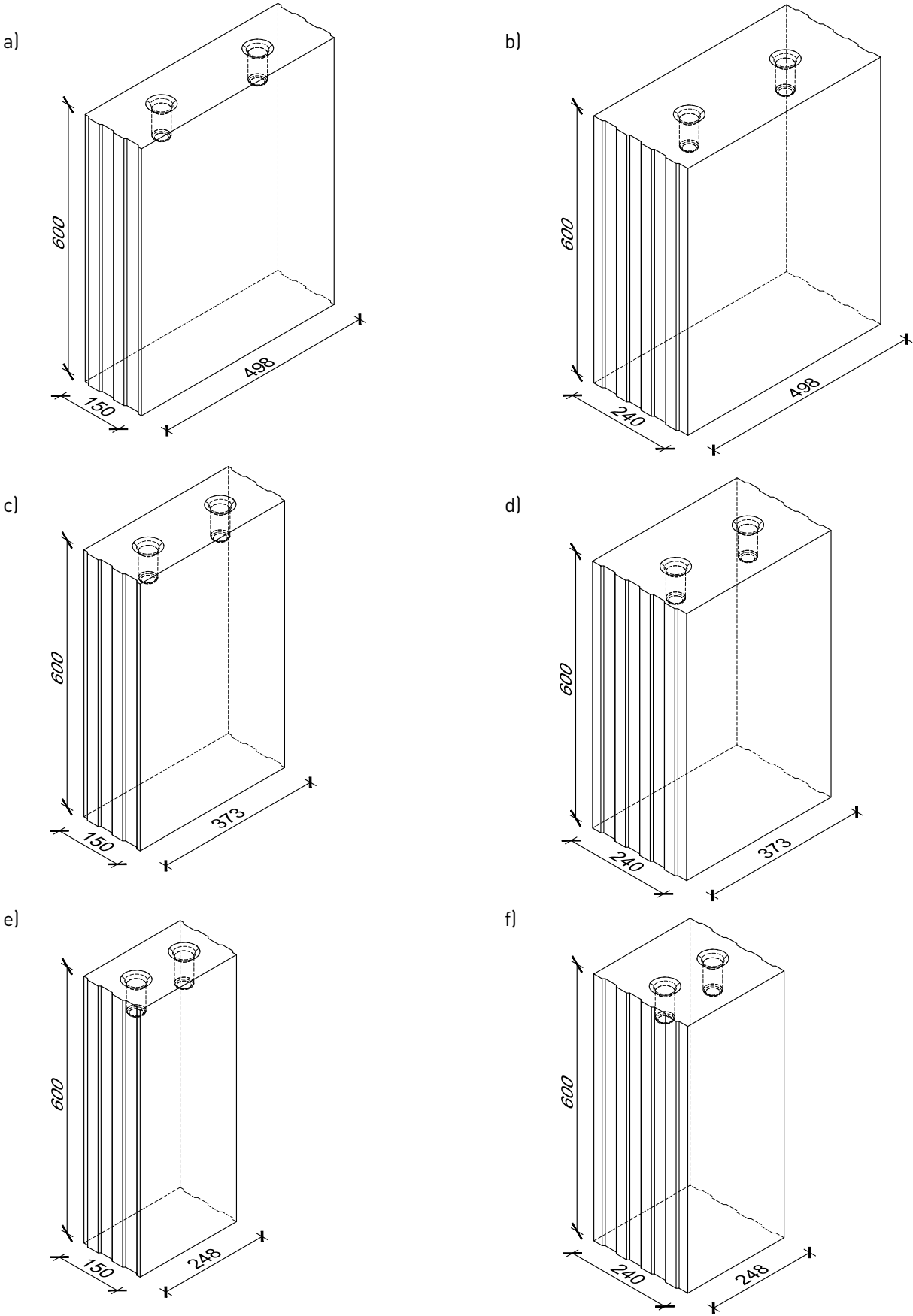
Rysunek 2.2. Elementy Silka Tempo, a) Silka Tempo 15, b) Silka Tempo 24, c) Silka Tempo 15 ¾, d) Silka Tempo 24 ¾, e) Silka Tempo 15 ½, f) Silka Tempo 24 ½
