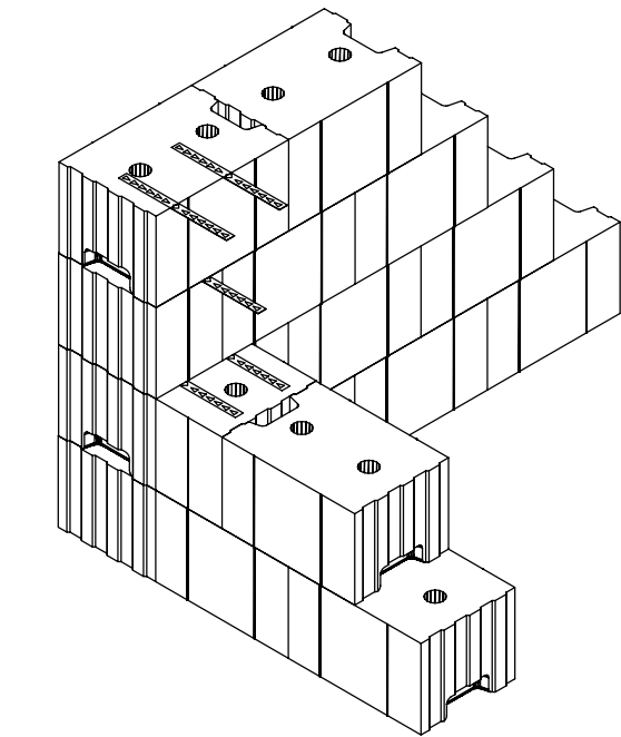
Rysunek 3.8. Łączenie ścian w narożu budynku za pomocą łączników LP30
