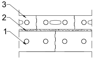
Rysunek 3.2. Ściana dwuwarstwowa wewnętrzna; 1 – blok Silka, 2 – spoina pionowa, 3 – blok Silka.
