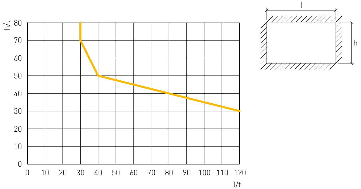
Wykres 3.1. Maksymalne wymiary ściany zamocowanej na czterech krawędziach
