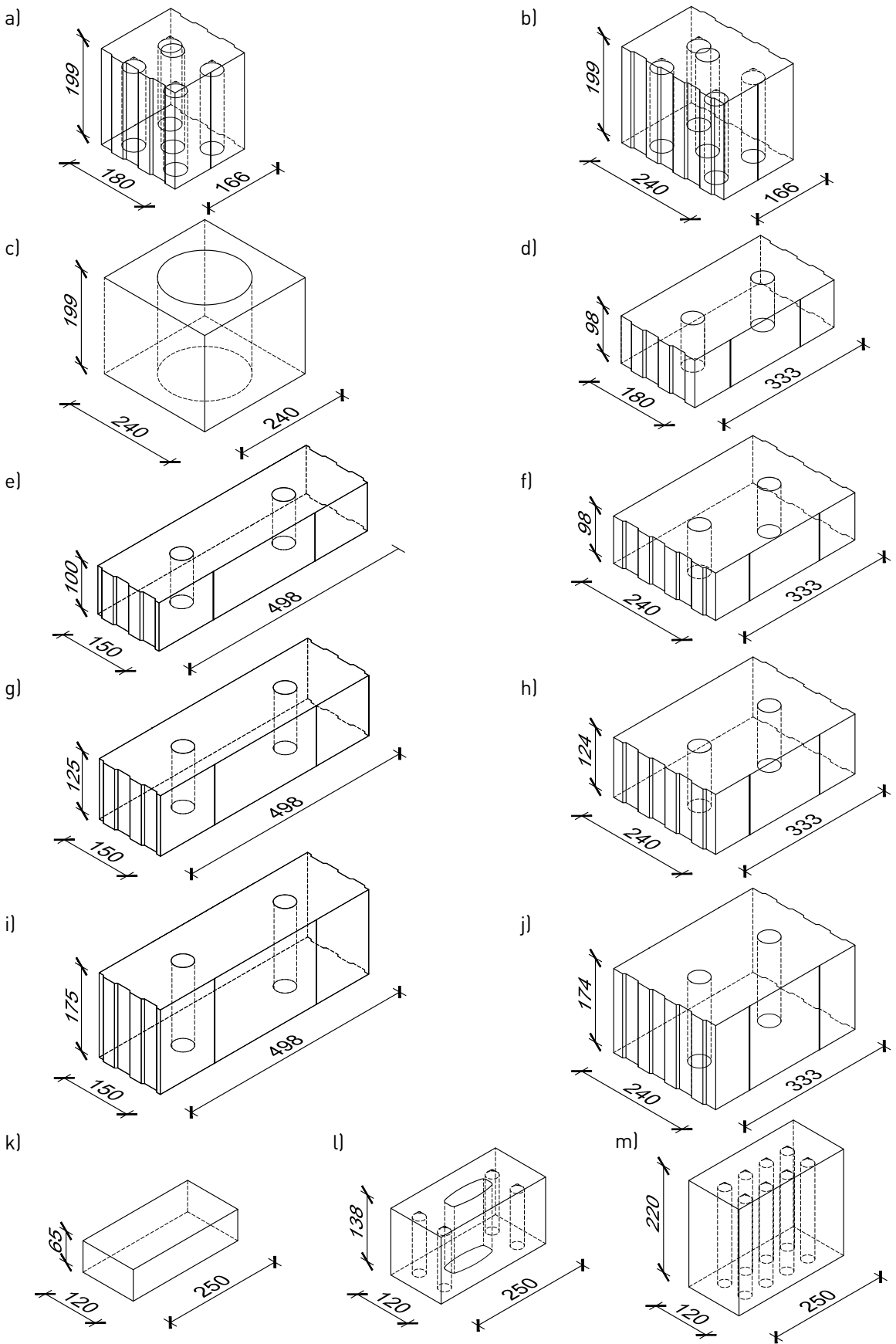
Rysunek 2.3. Elementy uzupełniające Silka: a) Silka ½ E18, b) Silka ½ E24, c) Silka EW, d) Silka EQ 10/18, e) Silka EQ 10/24, f) Silka EQ 10/24, g) Silka EQ 12,5/15, h) Silka EQ 12,5/24, i) Silka EQ 17,5/15, j) Silka EQ 17,5/24, k) Silka 1NF, l) Silka 2NFD, m) Silka 3NFD
